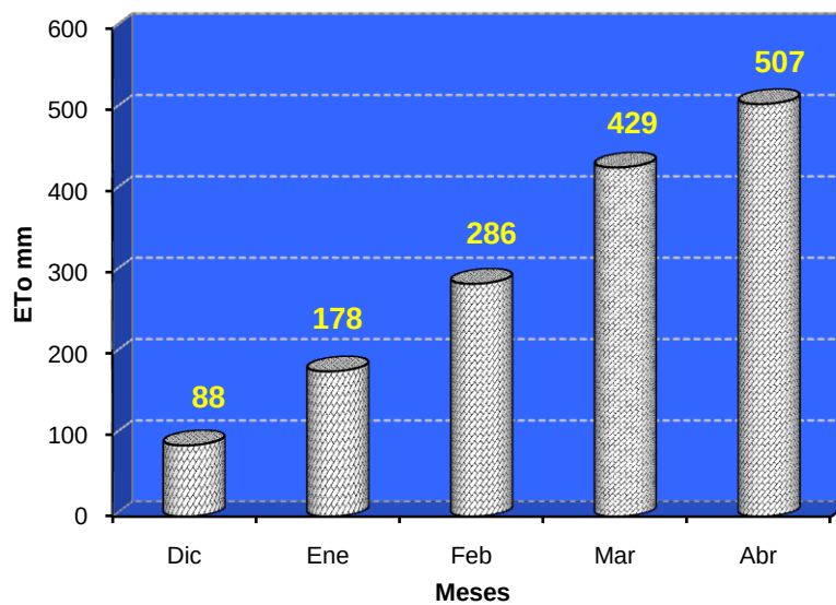
Figura 5. Valores de evapotranspiración en mm acumulados en el período 01/12/08 al 15/04/09
